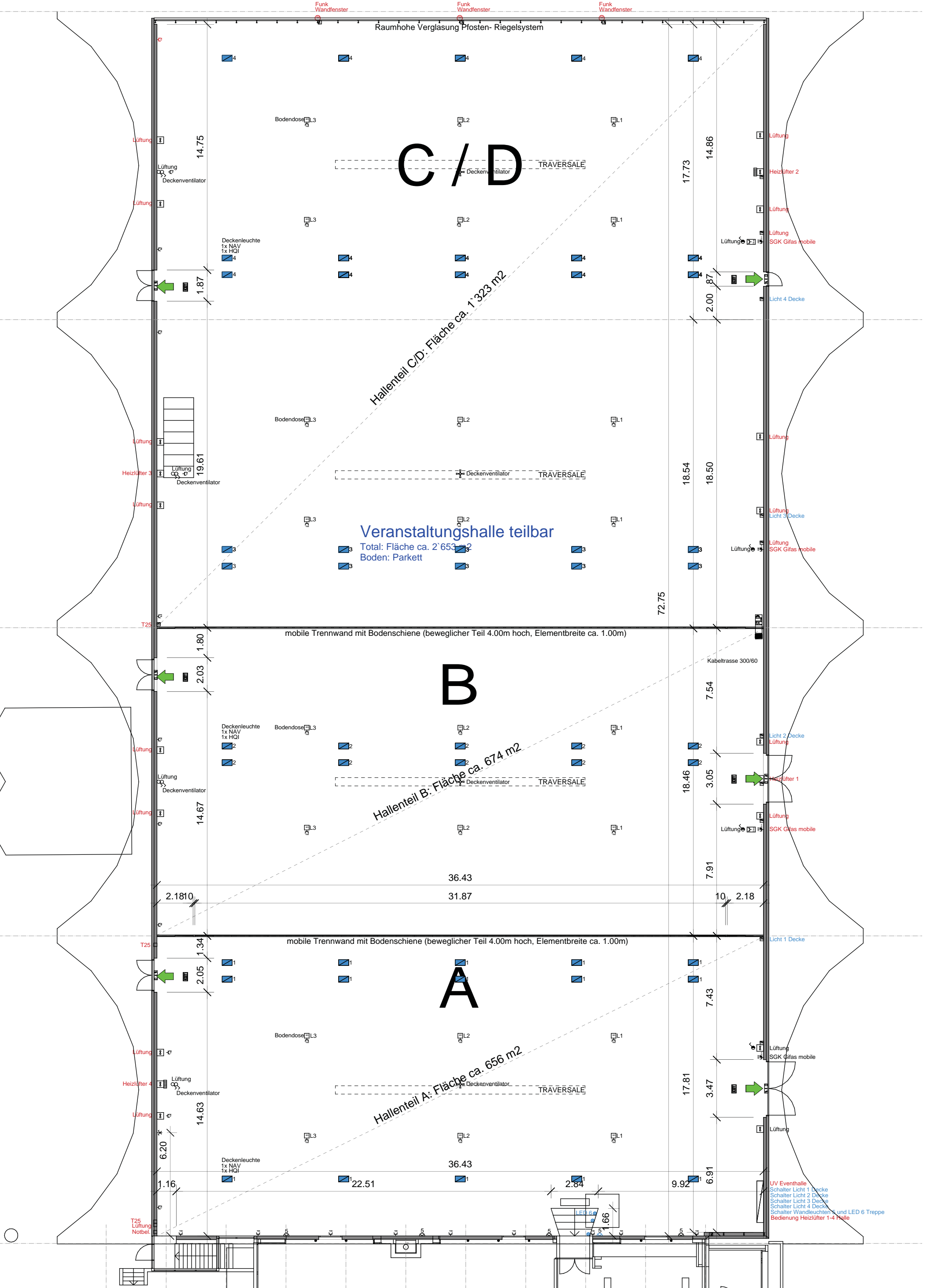
WESTHALLE PARKHOTEL LANGENTHAL GRUNDRISS 1:200
